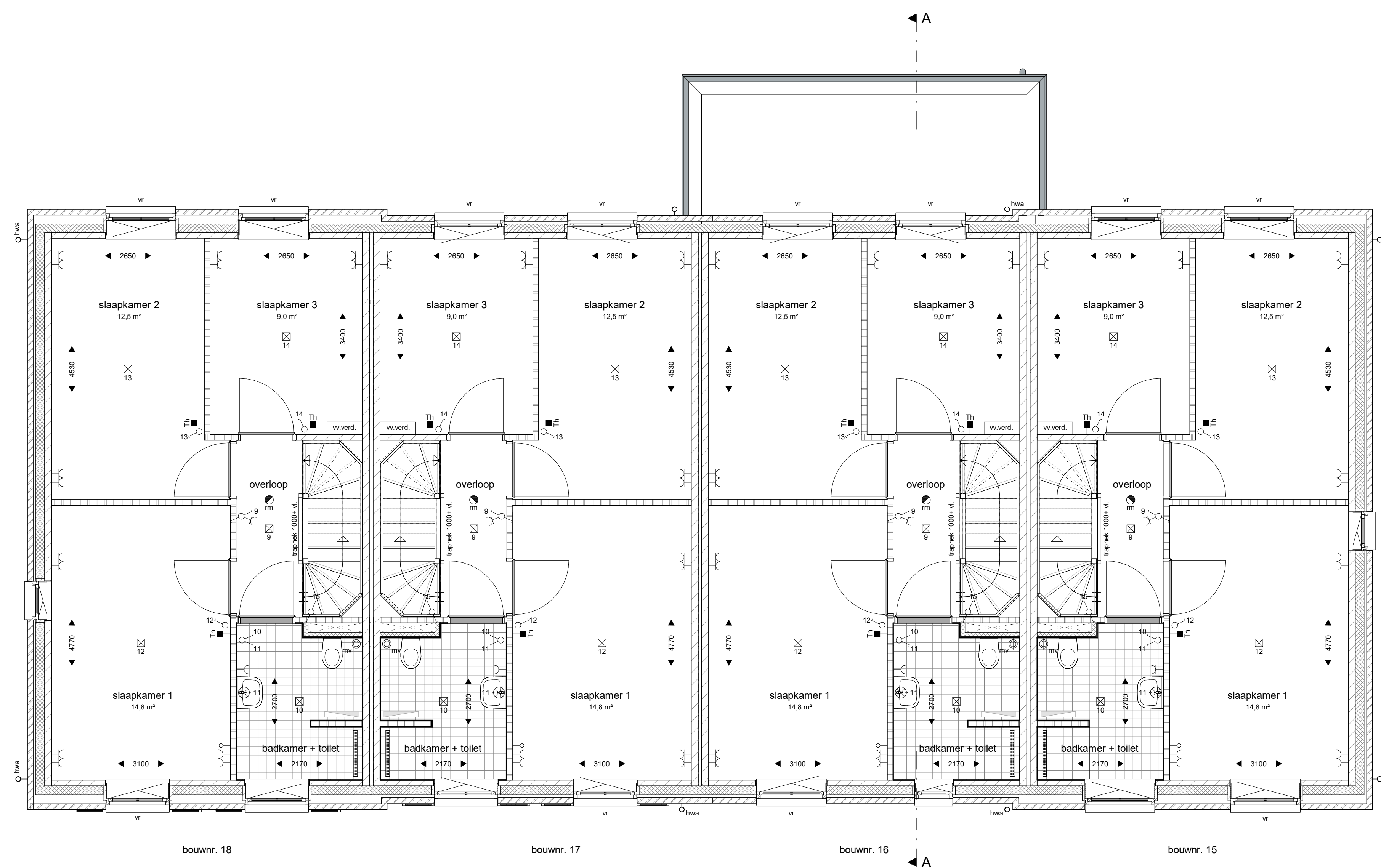
eerste verdieping 1 : 50
