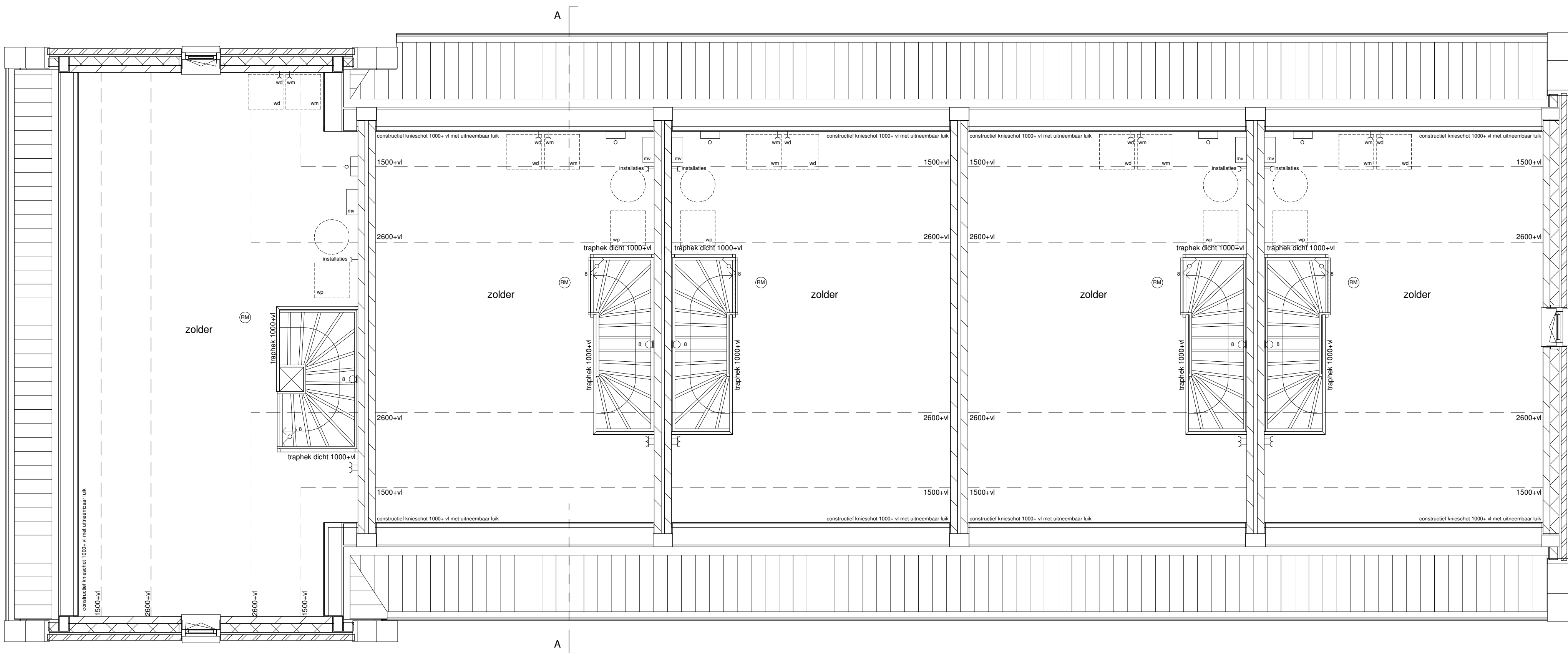
1: 50 tweede verdieping bouwnummer 05 type G bouwnummer 04 type H bouwnummer 03 type H bouwnummer 02 type H bouwnummer 01 type H
