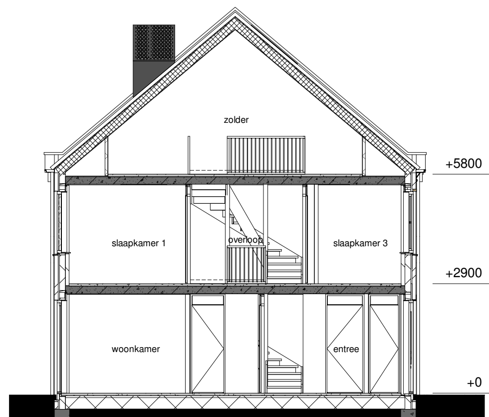
doorsnede AA
