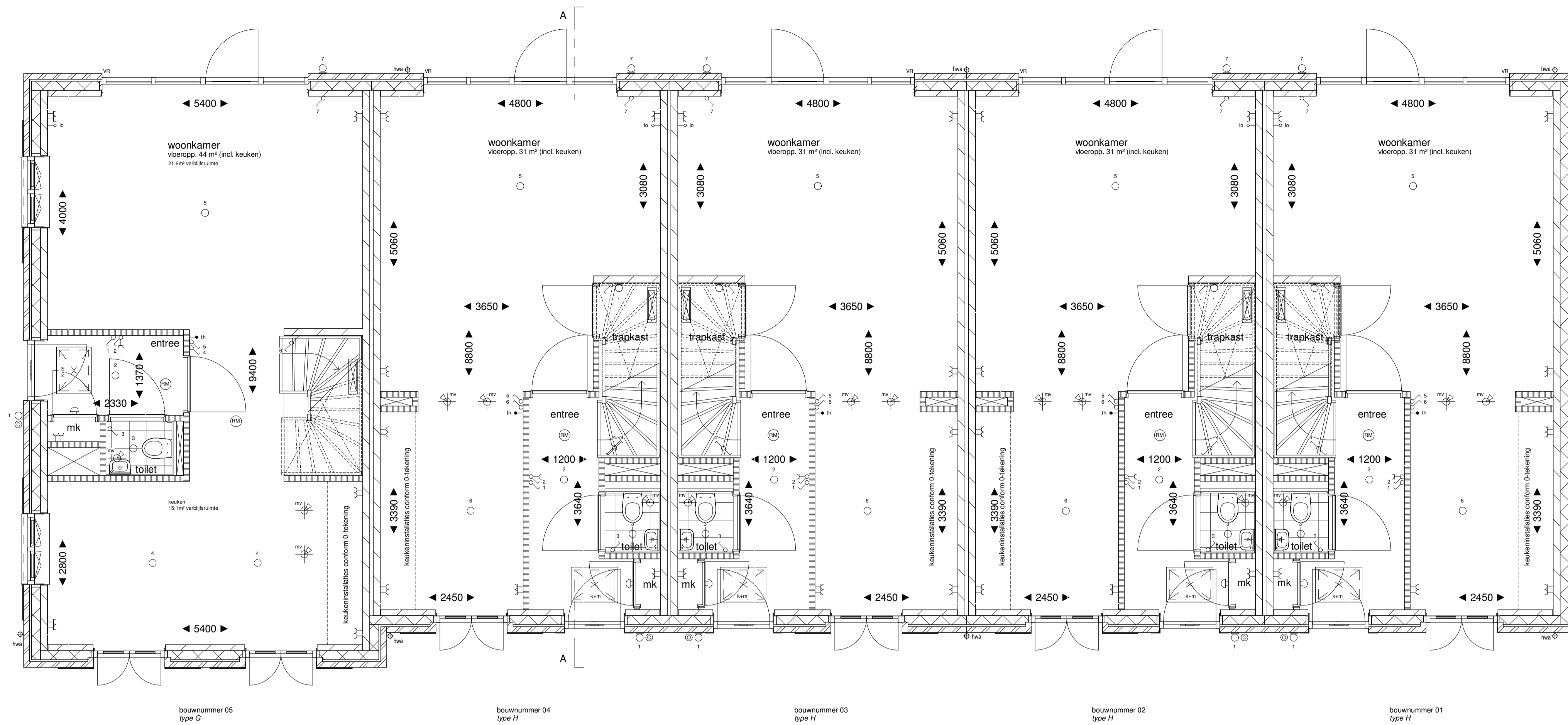
begane grond
