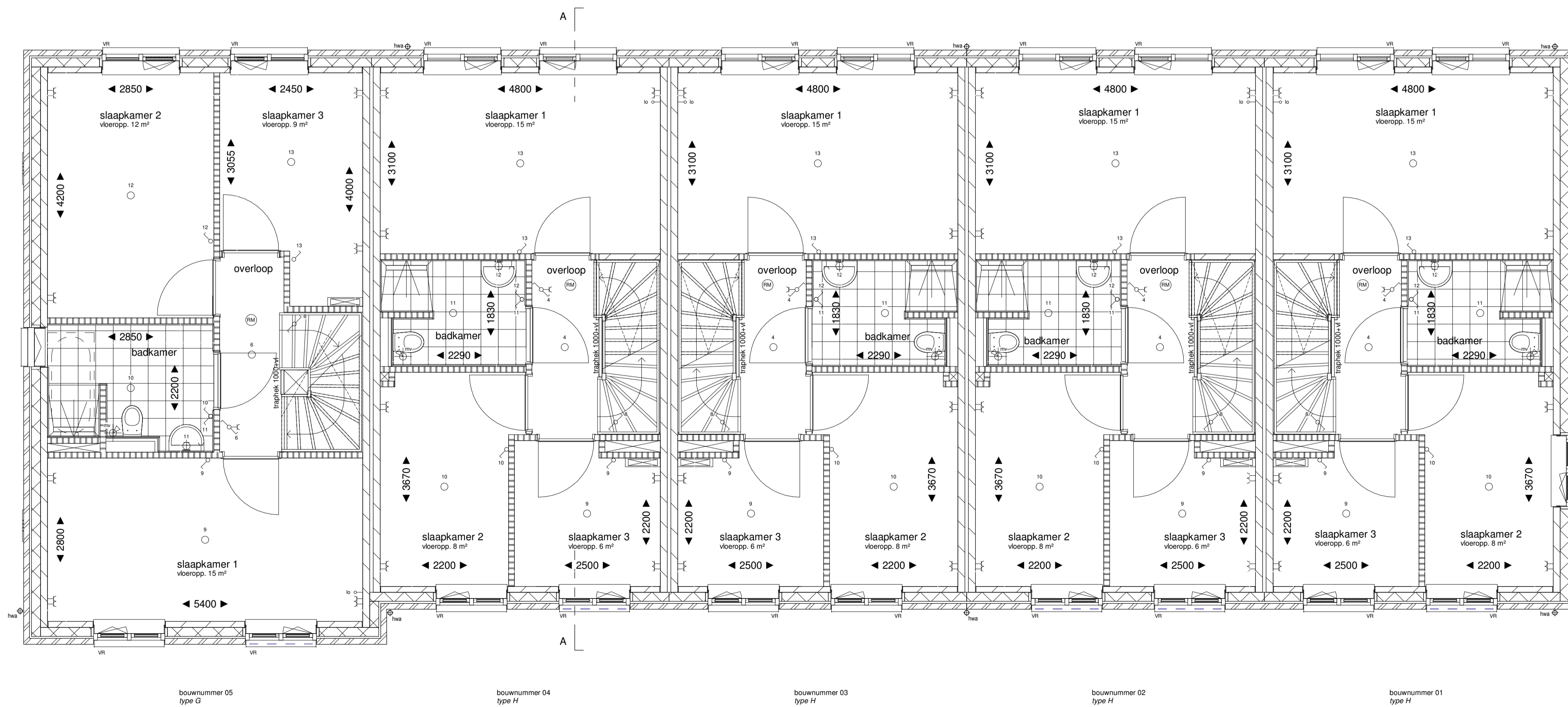
eerste verdieping
