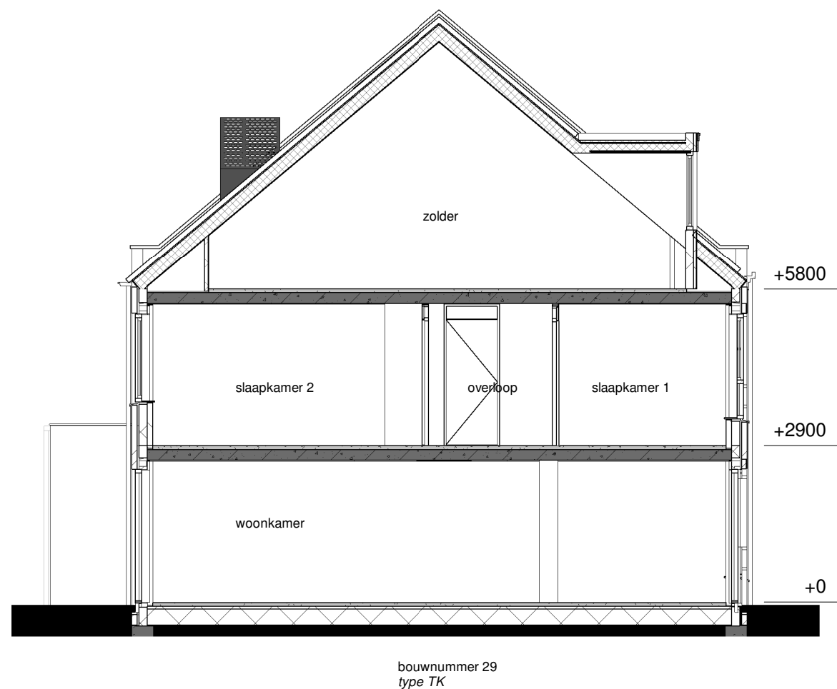
doorsnede KK
