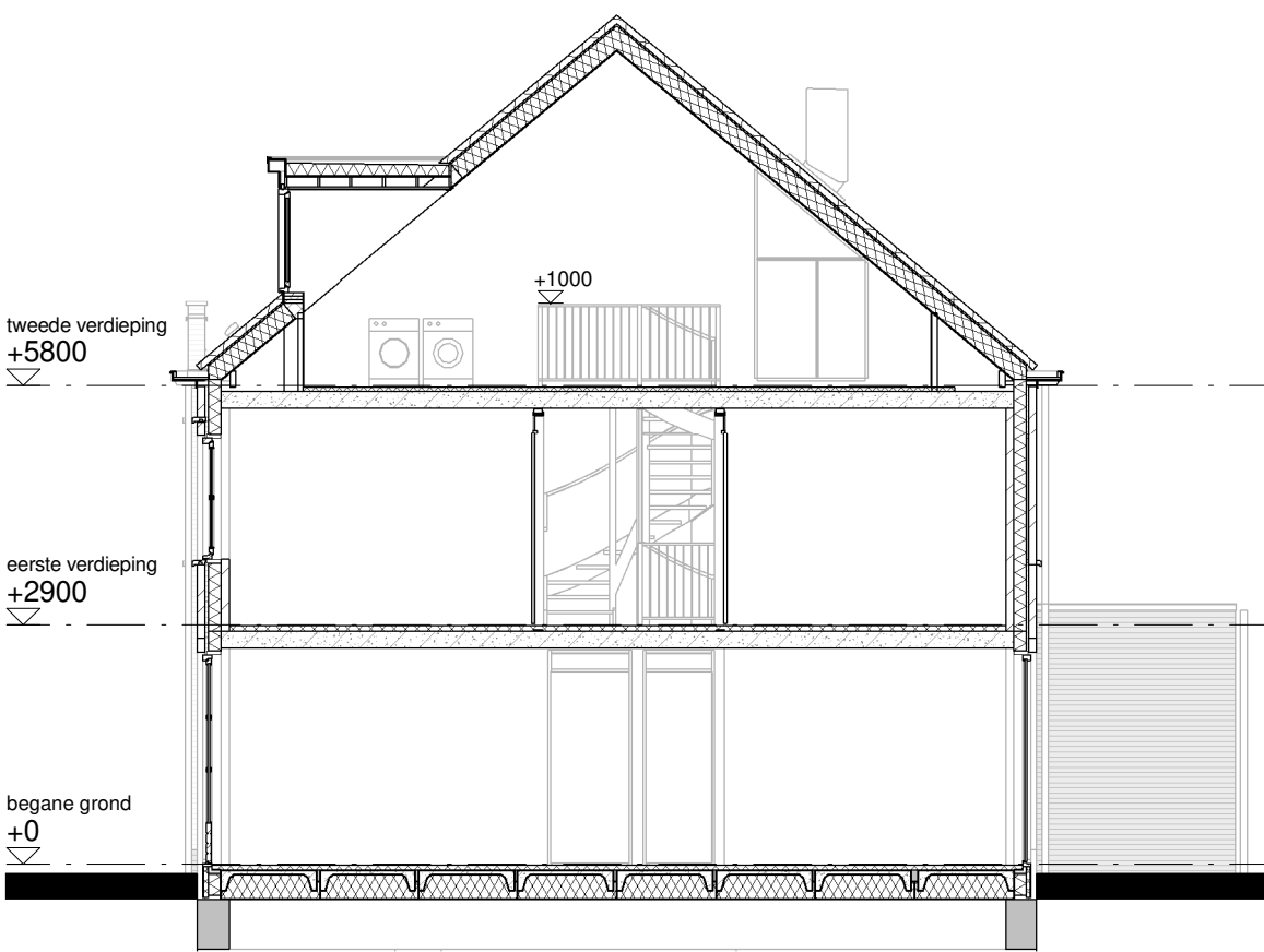
DOORSNED E A1 - A1 1:100
