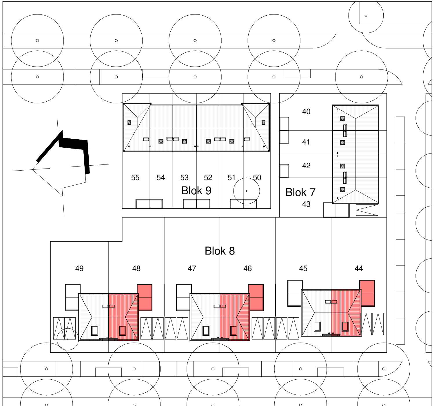
SITUATIE 1:500
