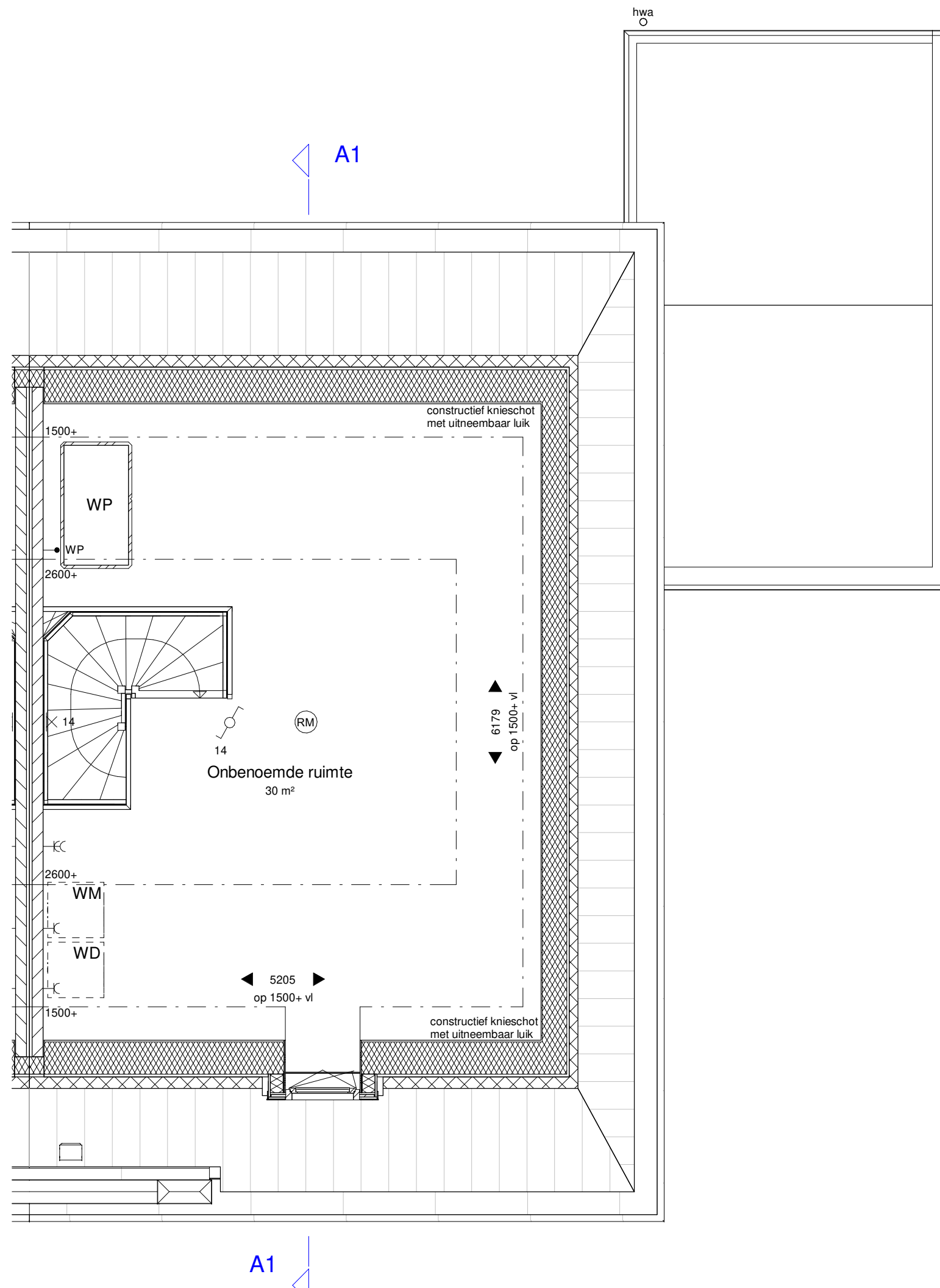
2de VERDIEPING 1:50
