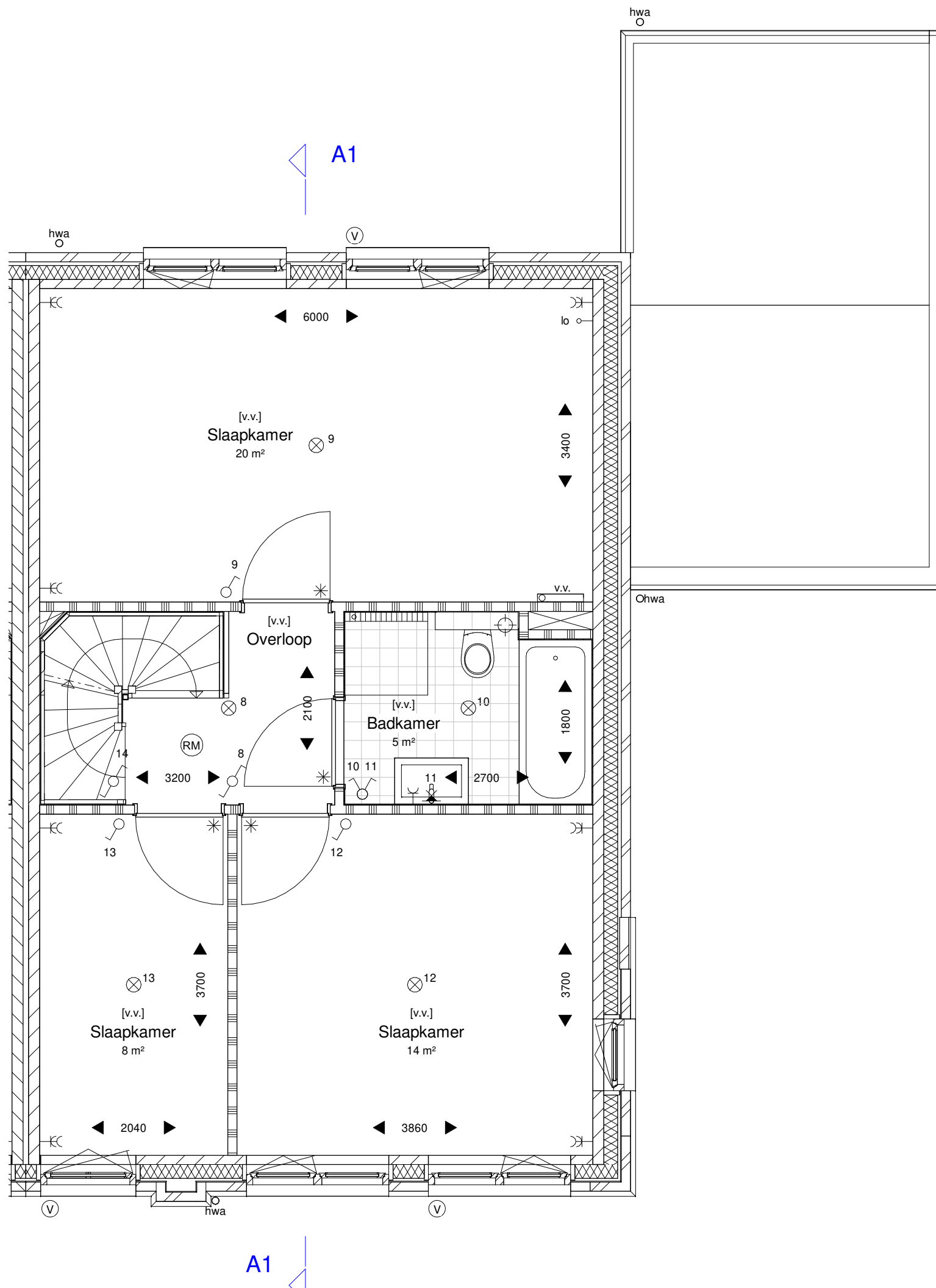
1ste VERDIEPING 1:50
