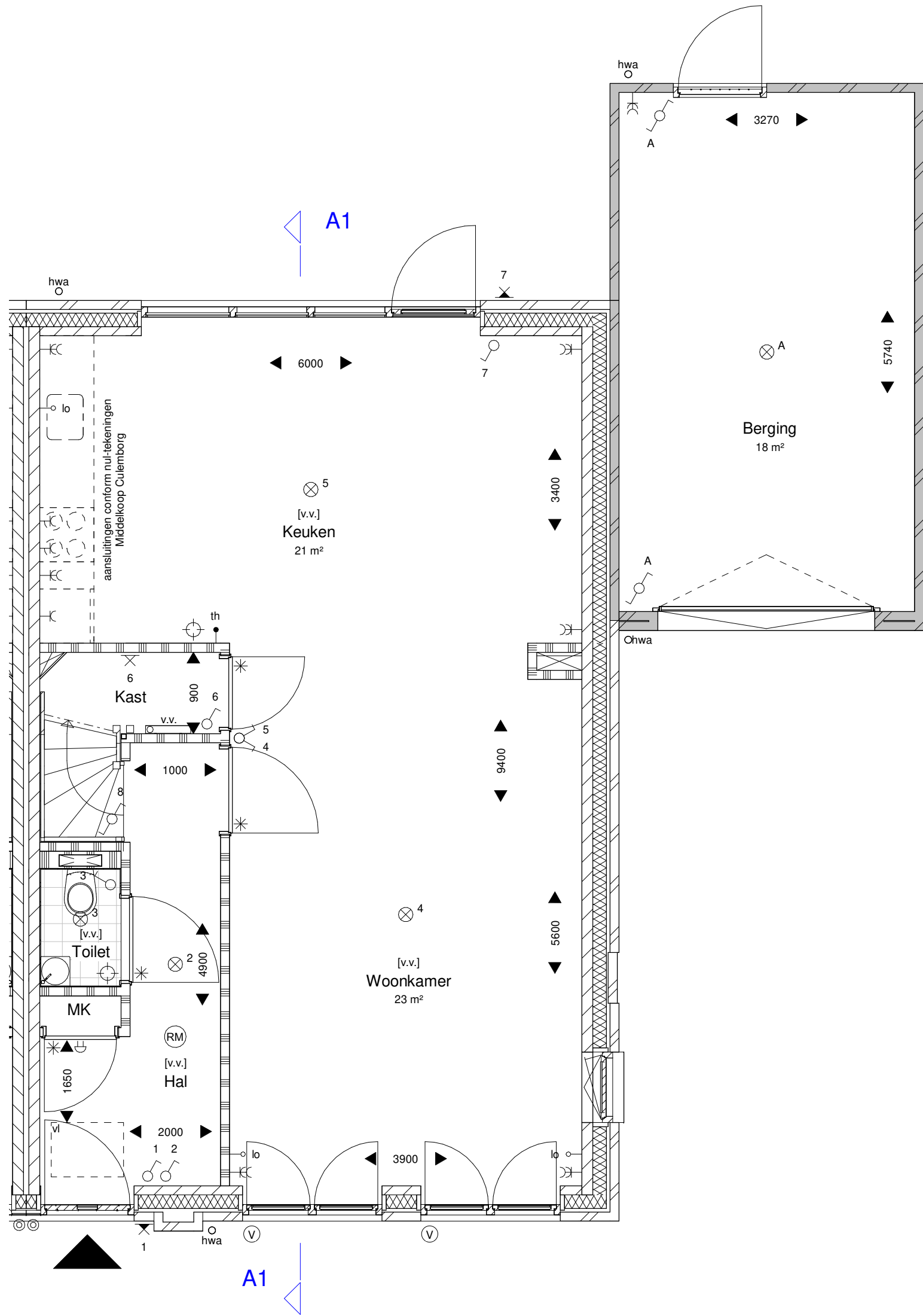
BEGANE GROND 1:50
