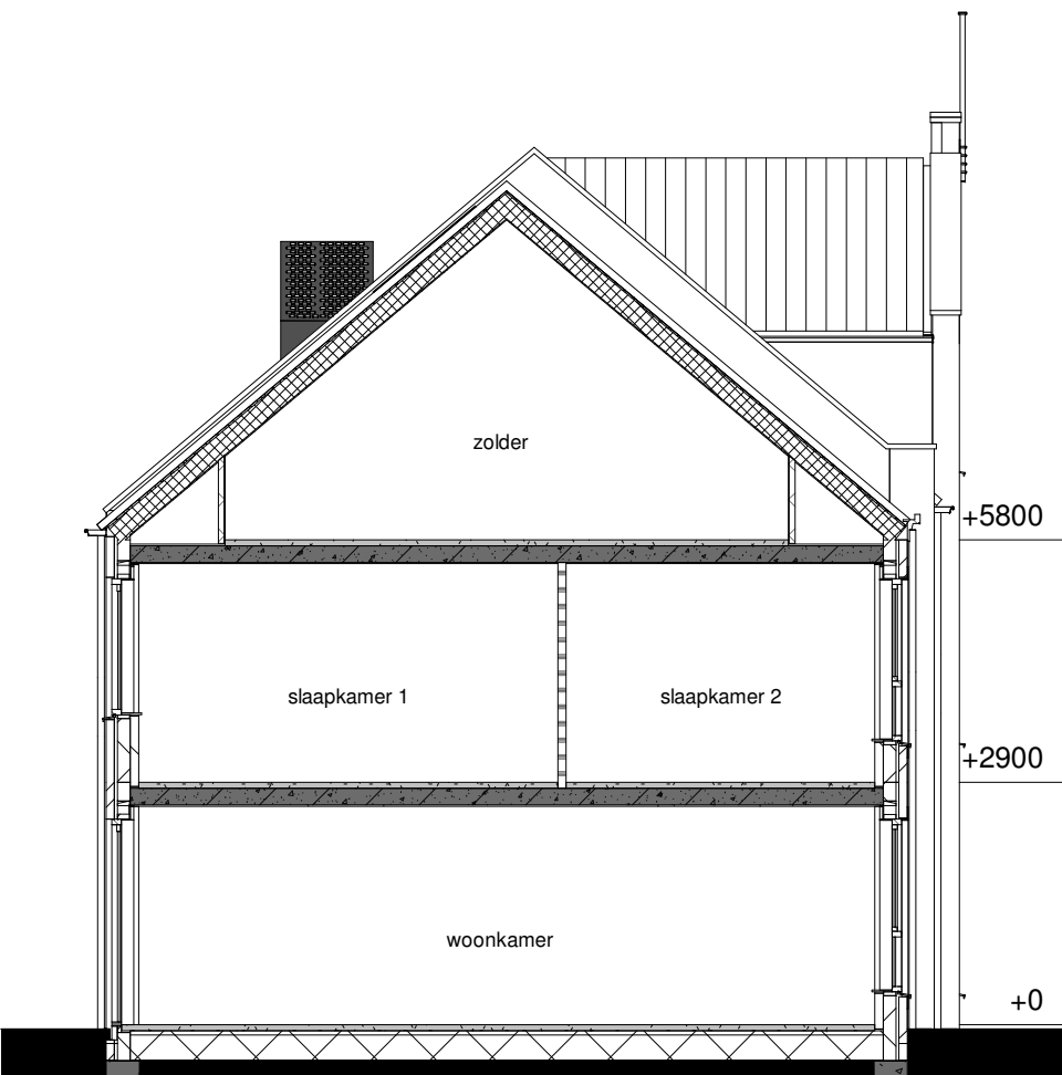
doorsnede CC
