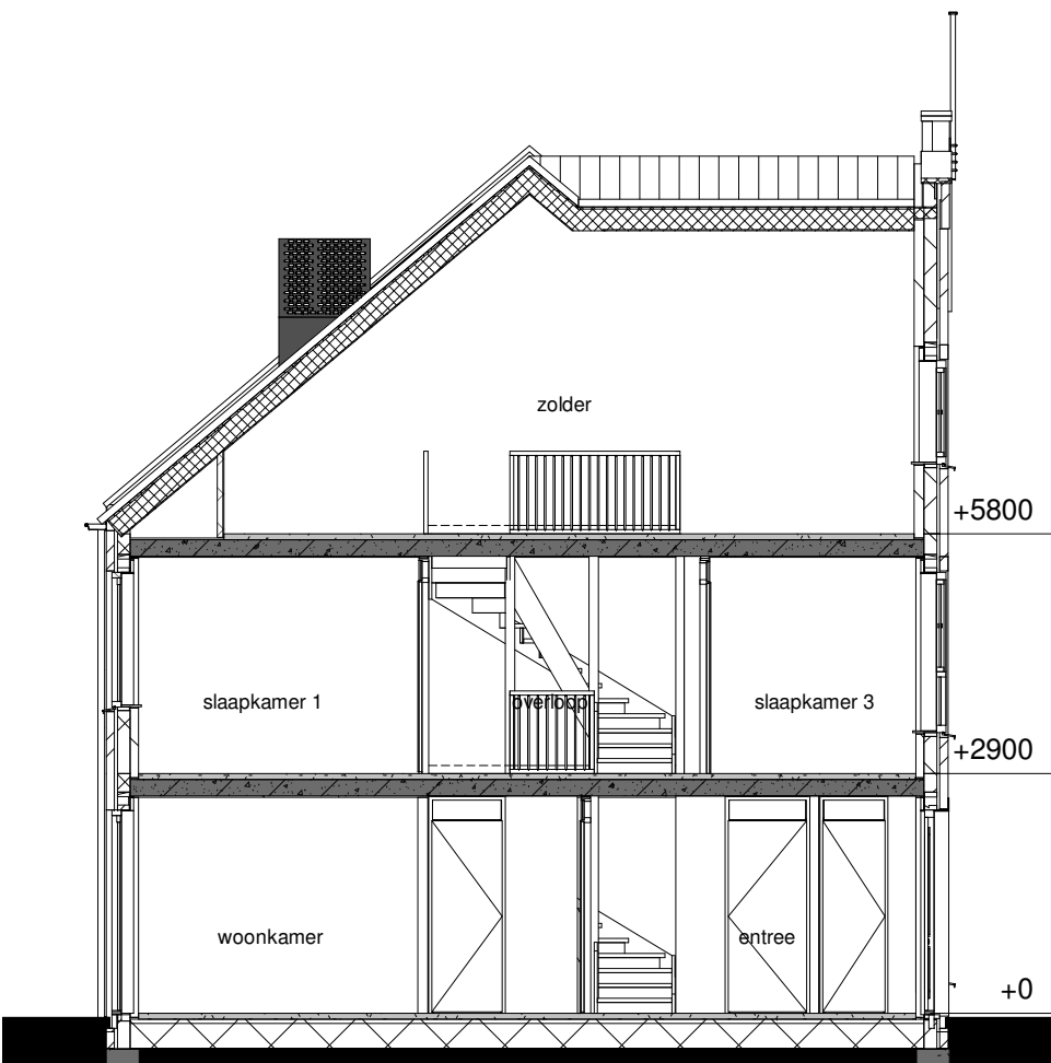
doorsnede DD
