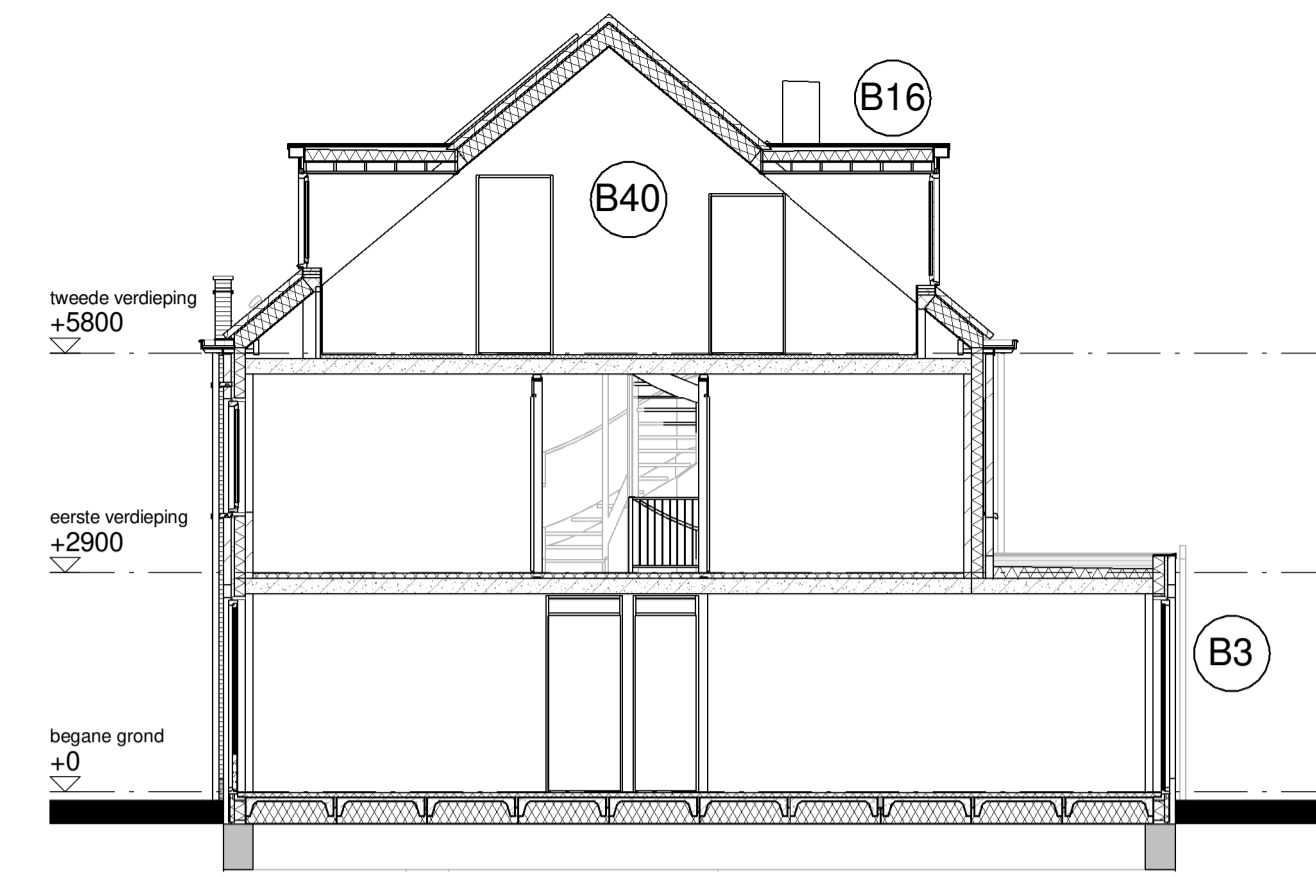
DOORSNEDE A2 - A2 1:100
