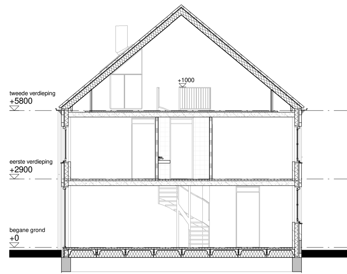
DOORSNEDE F7-F7 1:100
