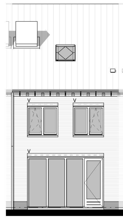
ACHTERGEVEL 1:100
