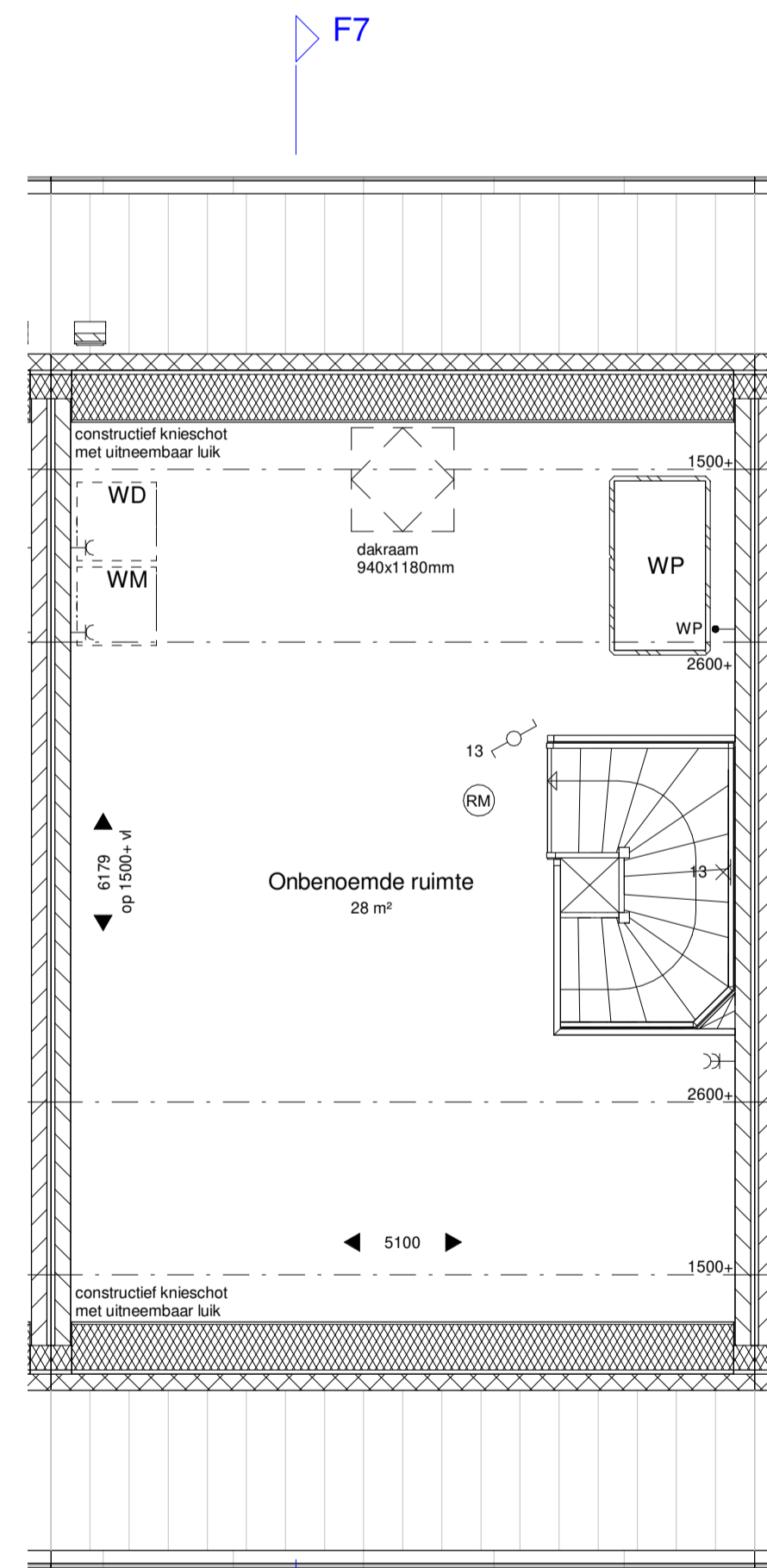
2de VERDIEPING 1:50
