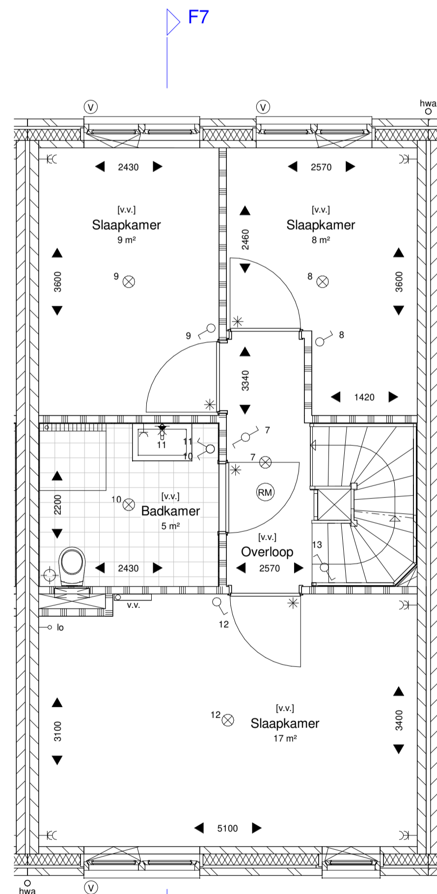
1ste VERDIEPING 1:50
