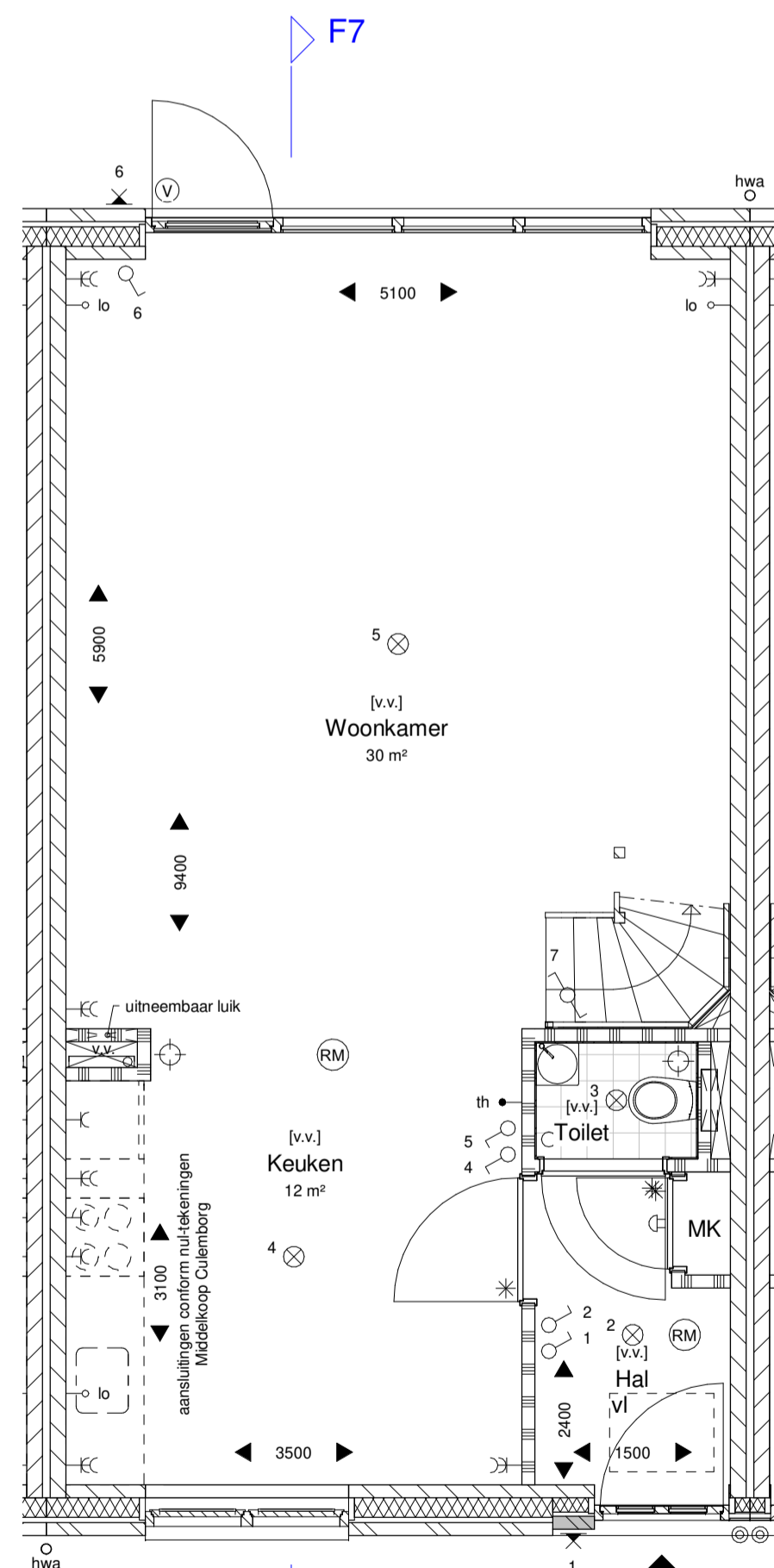
BEGANE GROND 1:50
