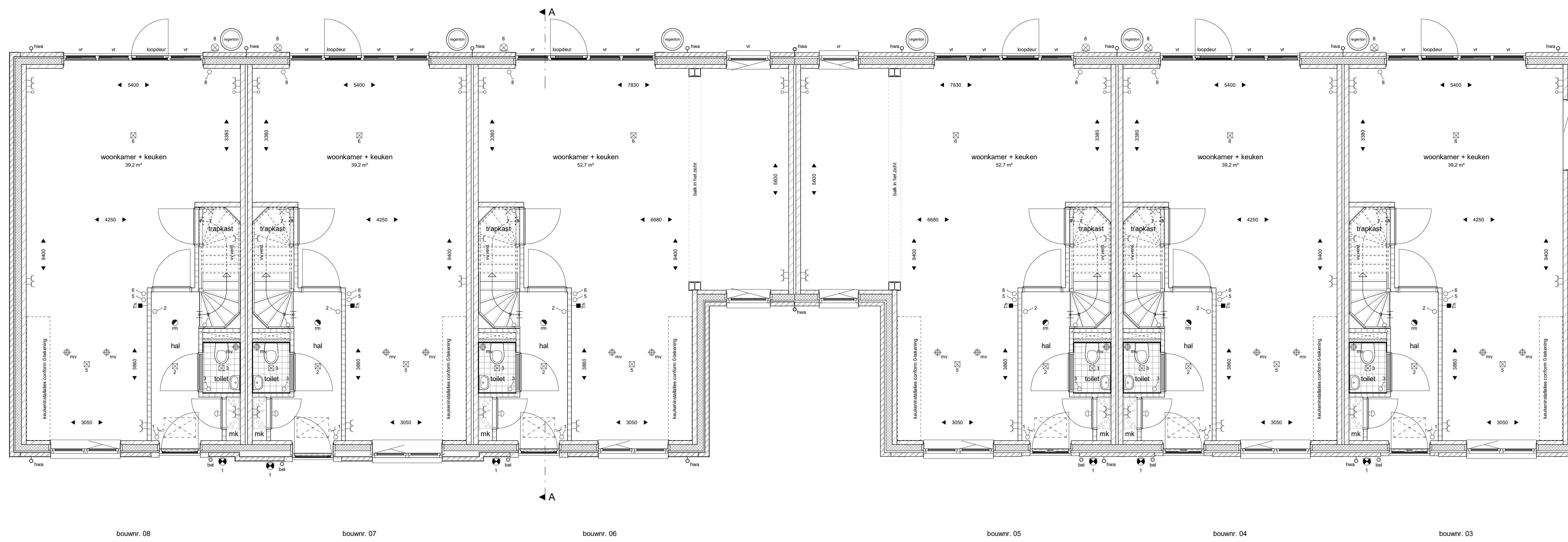
begane grond 1 : 50
