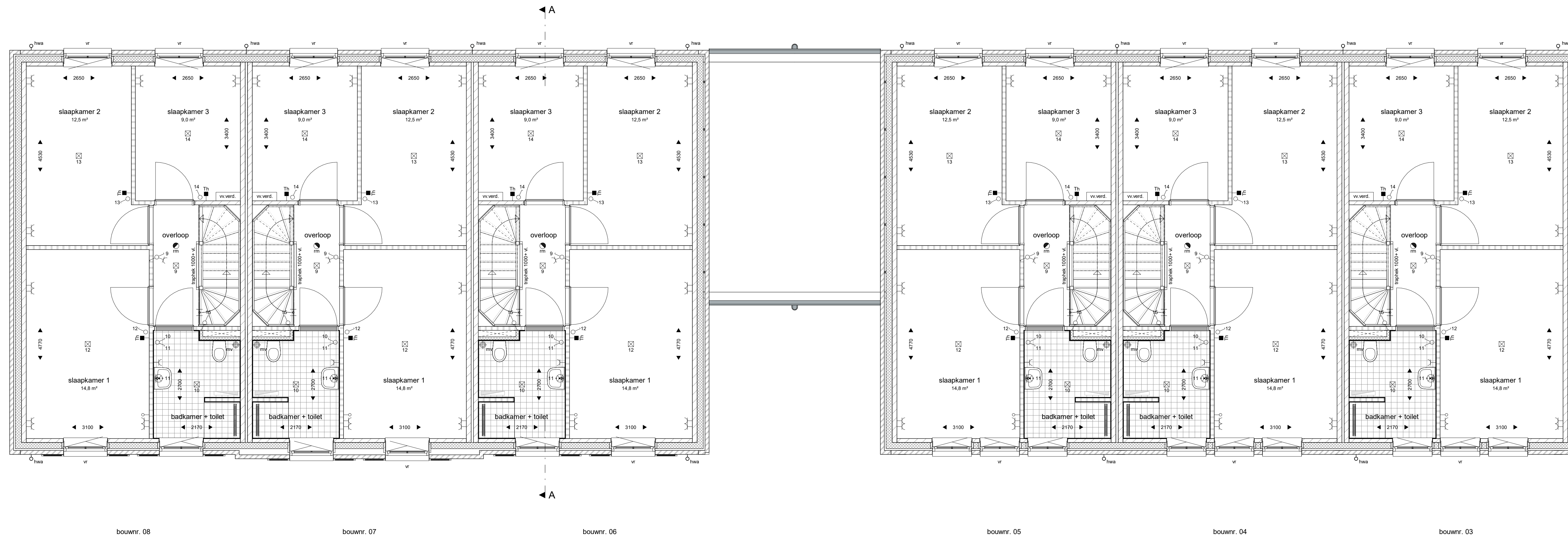
eerste verdieping 1 : 50
