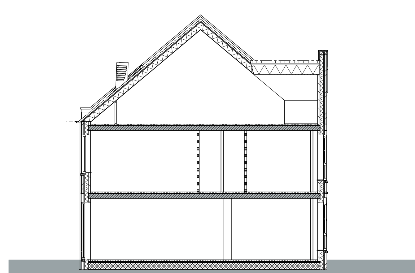
doorsnede B5-B5 1 : 100
