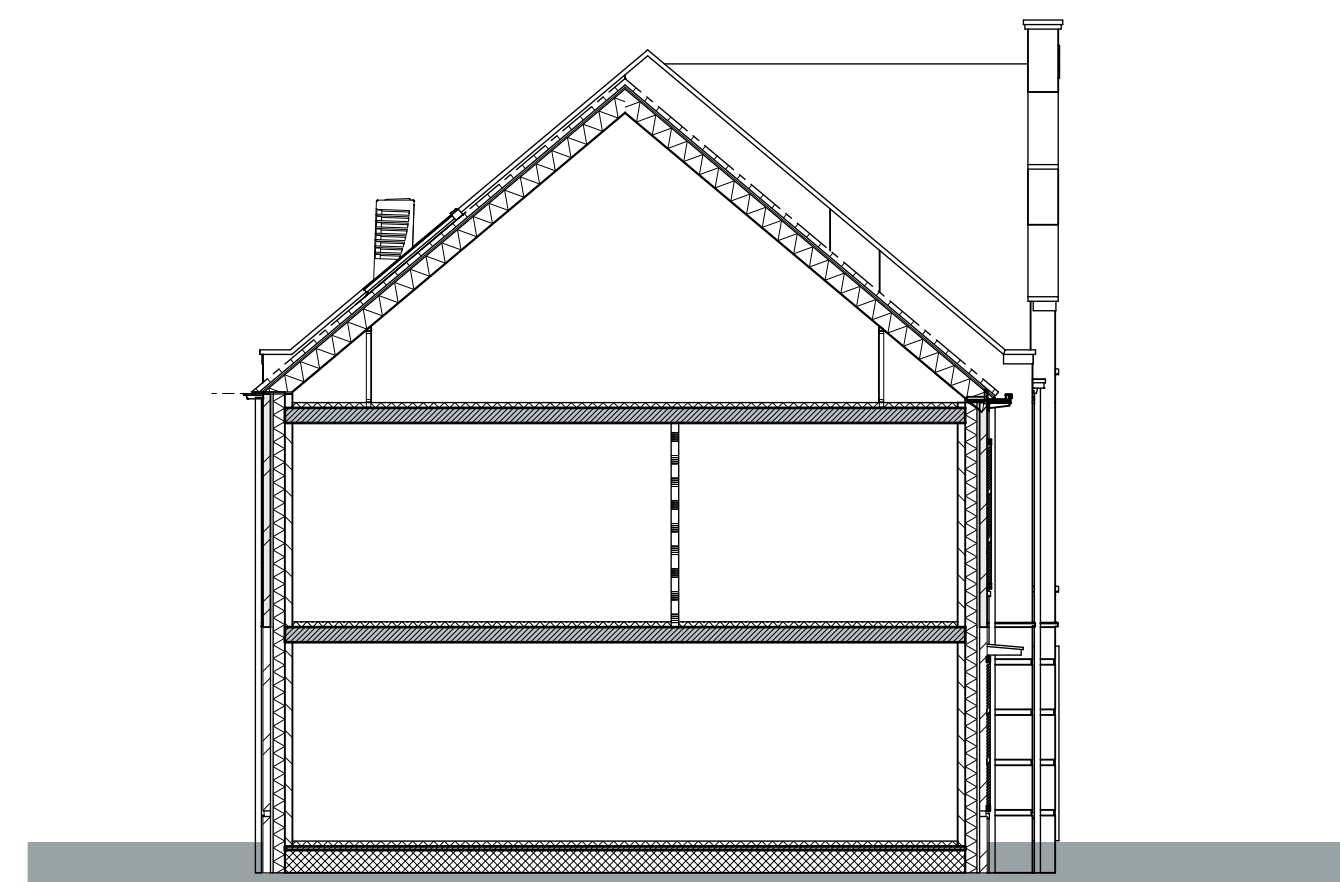
doorsnede A5-A5 1 : 100
