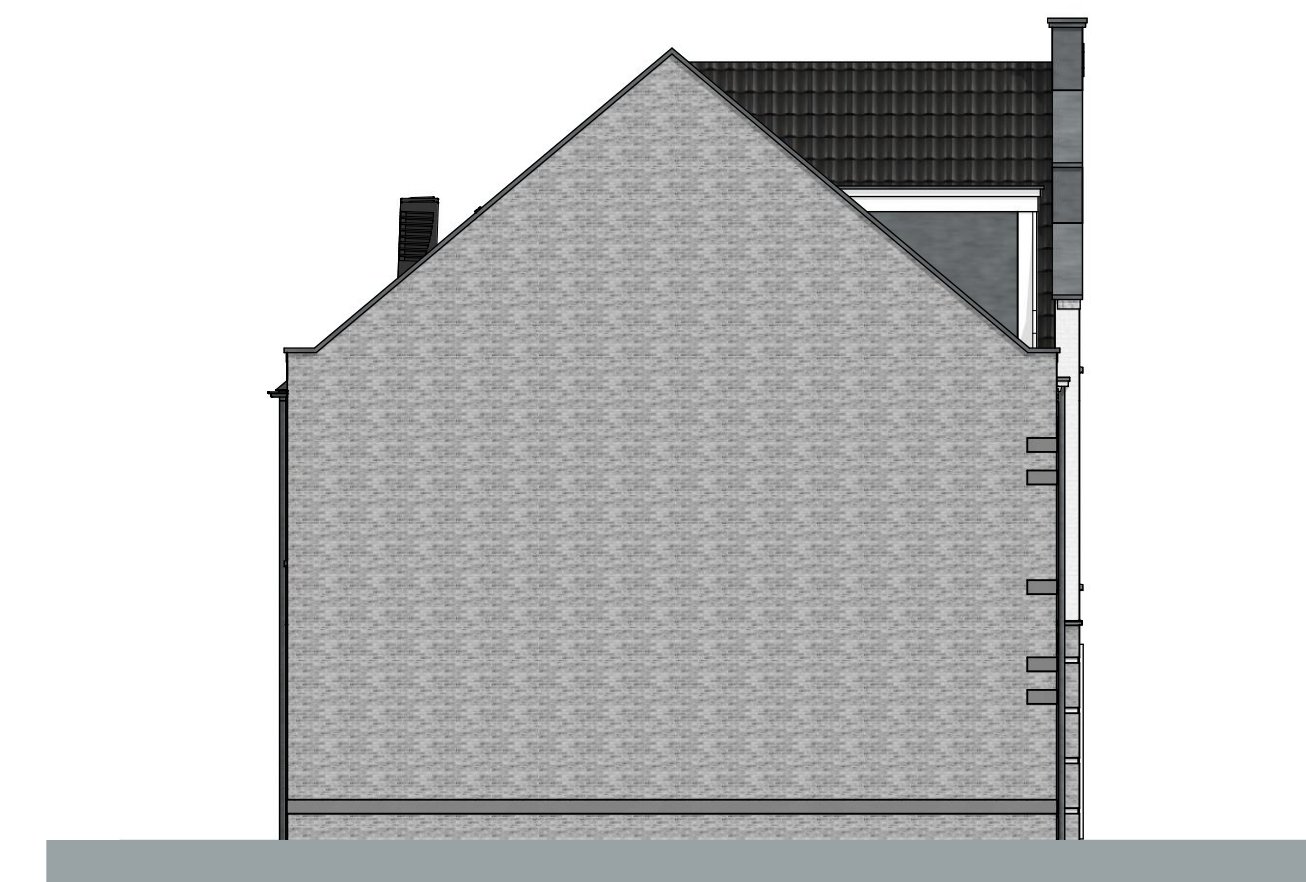
linkergevel 1 : 100
