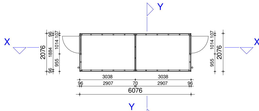
BEGANE GROND
