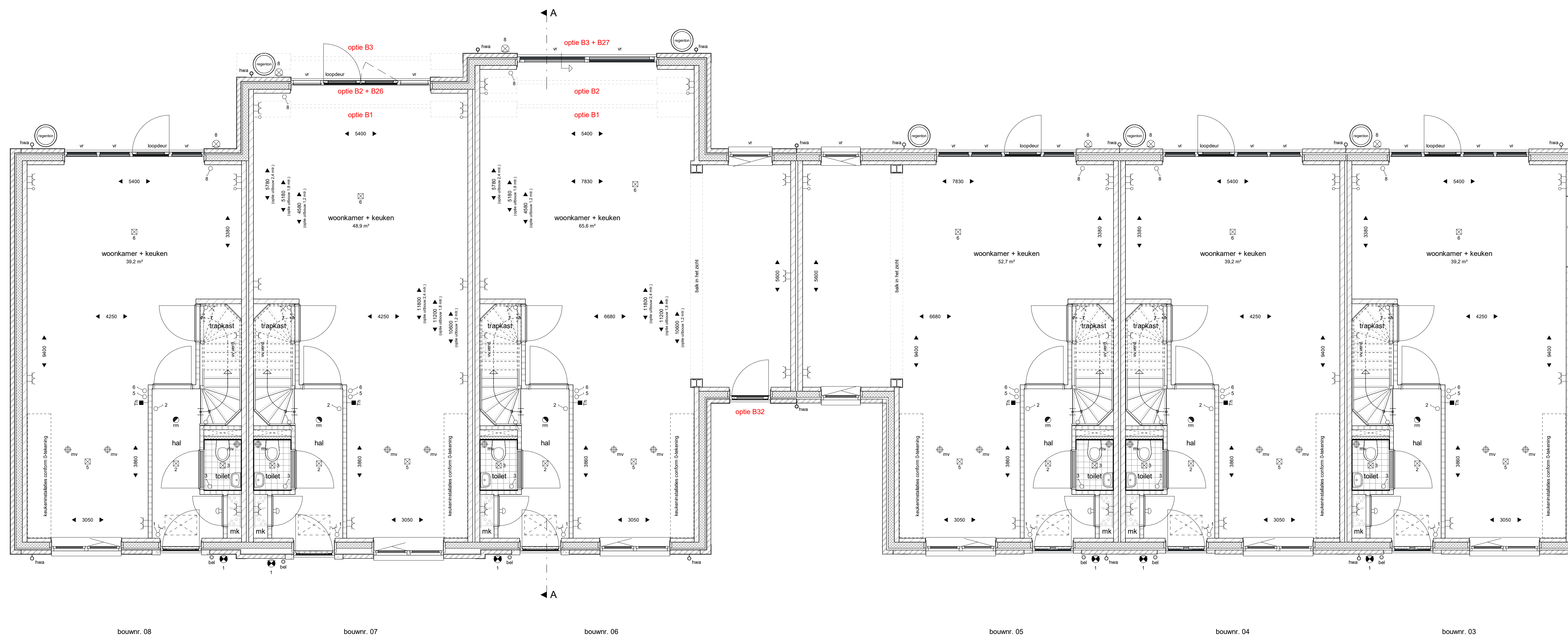
begane grond 1 : 50
