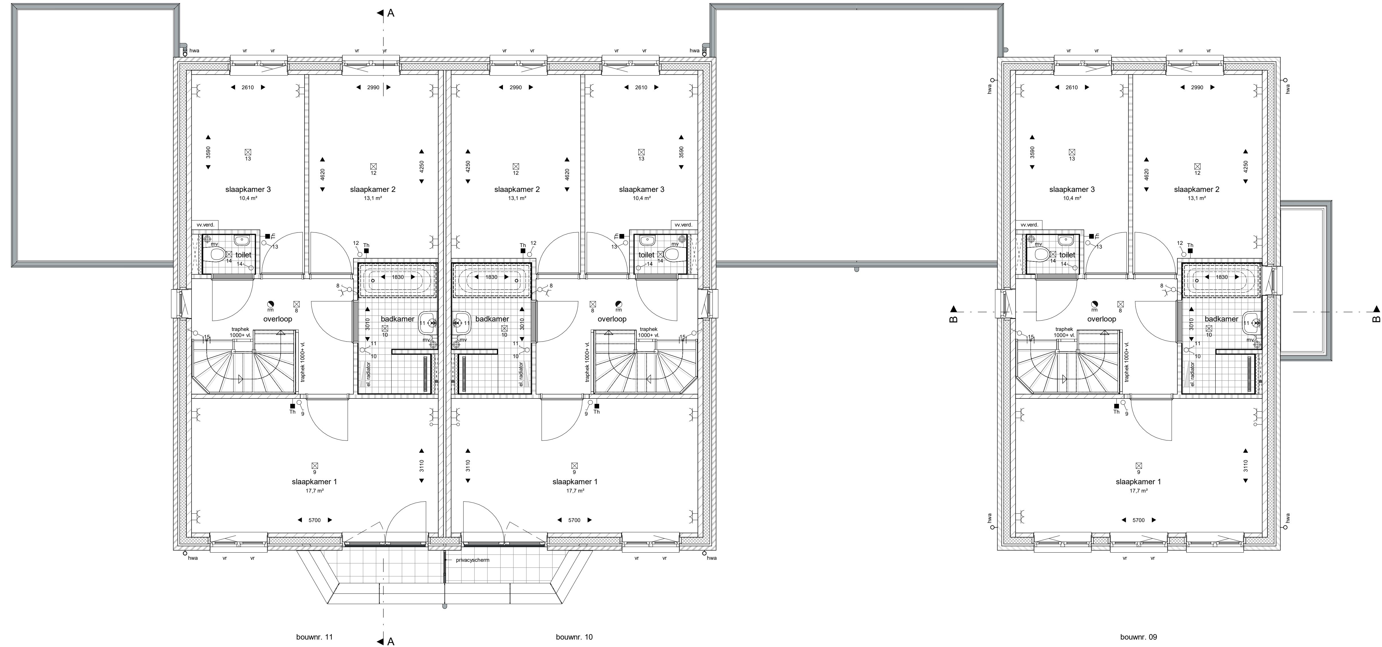
eerste verdieping 1 : 50
