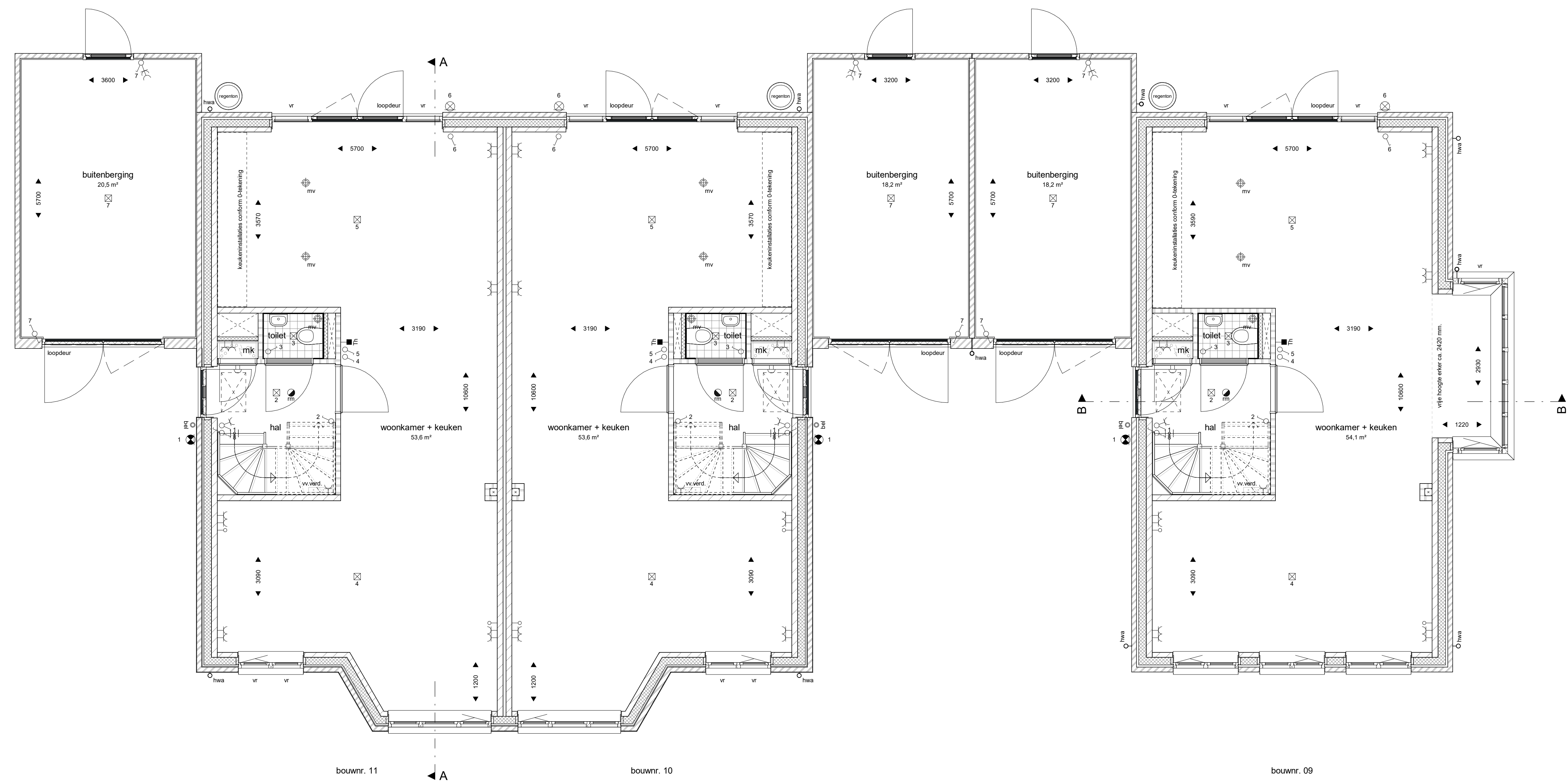
begane grond 1 : 50
